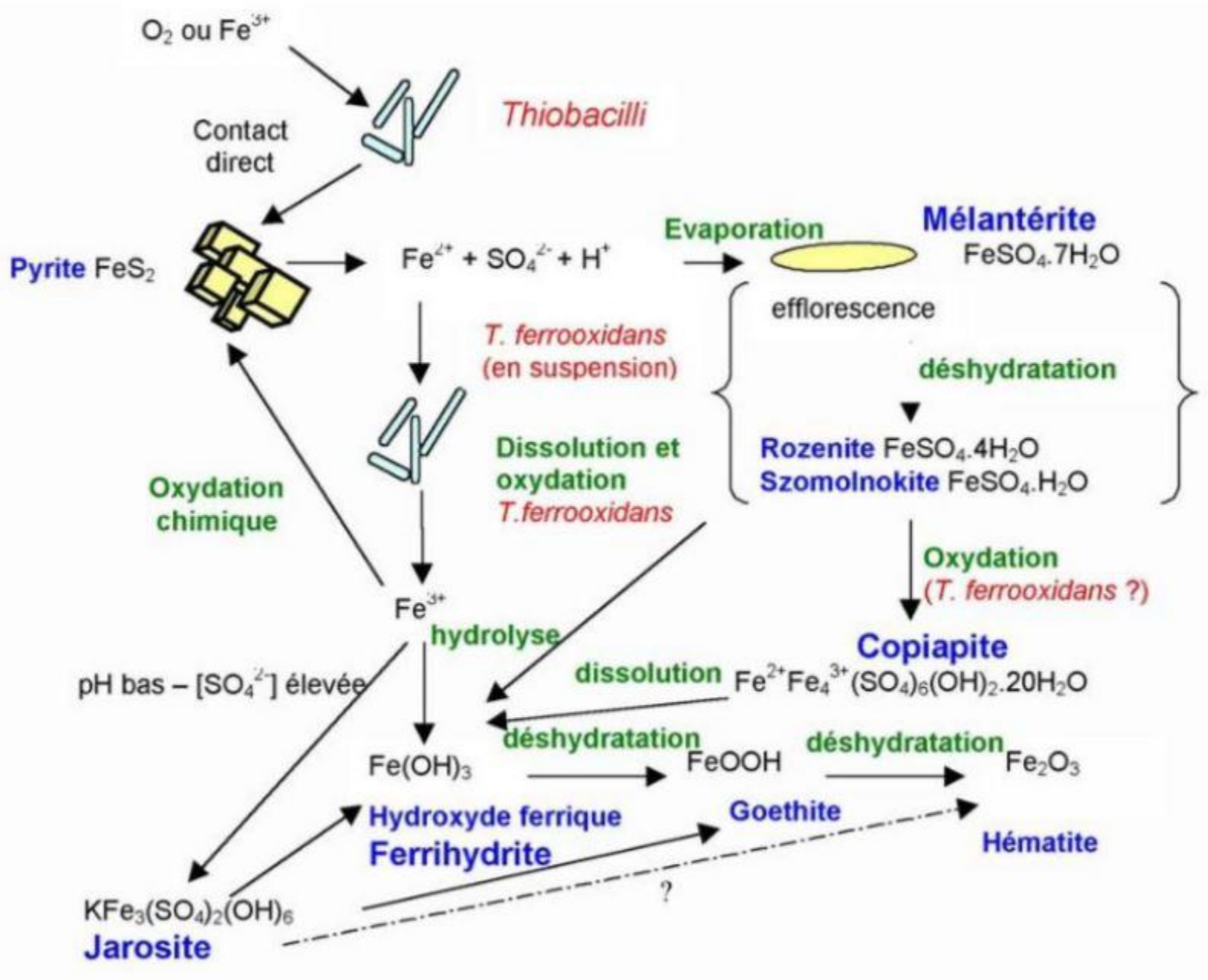
Figure 3 : Schéma récapitulatif des réactions primaires et secondaires se déroulant au cours d'un phénomène de DMA, d'après Nordstrom [1982].
